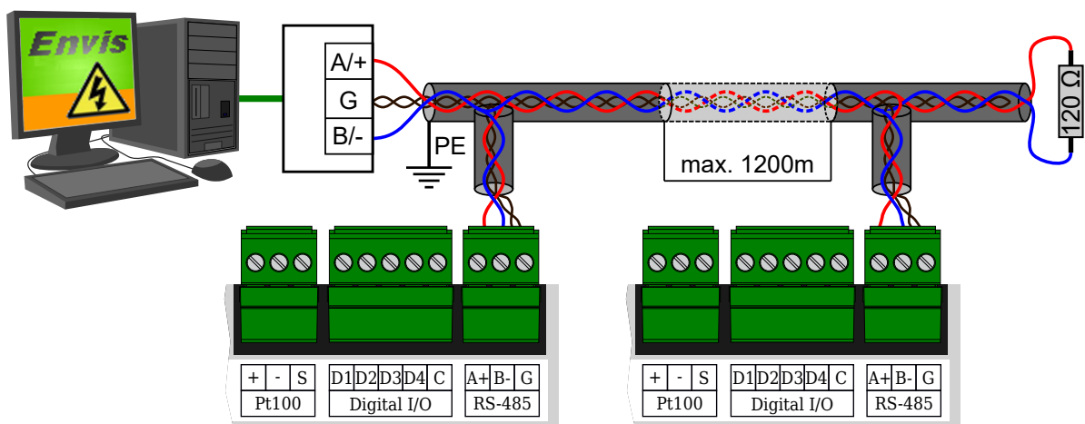
Obrázek 8: Zapojení komunikačních linek sběrnice RS-485 přístrojů ARTIQ 233.
