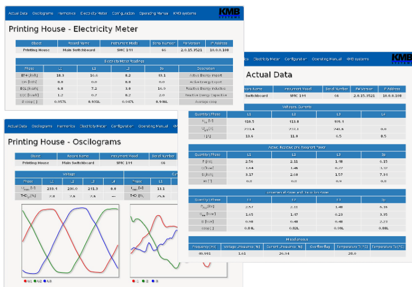
Obrázek 33: Zobrazení aktualních dat, elektroměru a oscilogramů na webové stránce přístroje.
