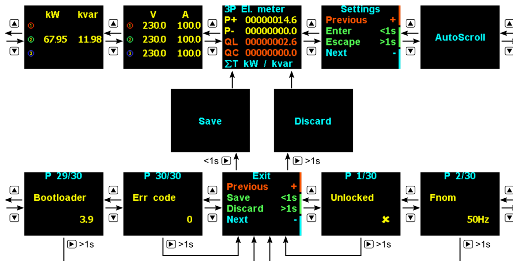
Obrázek 13: Odchod z nastavení. Z nastavení je možné odejít pouze přes obrazovku Exit , kterou je možné nalistovat tlačítka nahoru/dolů, nebo využít funkci Escape (stisk prostředního tlačítka na déle než 1 s). Při krátkém stisku prostředního tlačítka (kratším než 1 s) na obrazovce Exit se provede uložení a uplatnění všech změn v nastavení, což je po dobu 2 s indikováno obrazovkou Save . V tuto chvíli může dojít k restartu přístroje, pokud došlo například ke změně Fnom . Při dlouhém stisku prostředního tlačítka (delším než 1 s) na obrazovce Exit dojde k zahození všech změn, což je indikováno po dobu 2 s obrazovkou Discard , obrazovka se přepne zpět do smyčky obrazovek aktuálních dat a přístroj běží beze změn dále.
