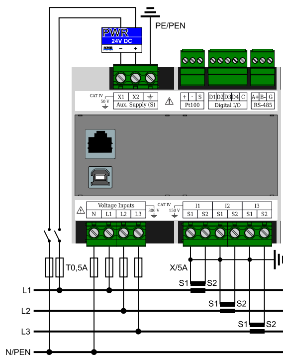
Obrázek 6: Příklad typického zapojení přístroje ARTIQ 233 v síti NN — zapojení měřeného napětí do hvězdy ve čtyřvodičové síti.
