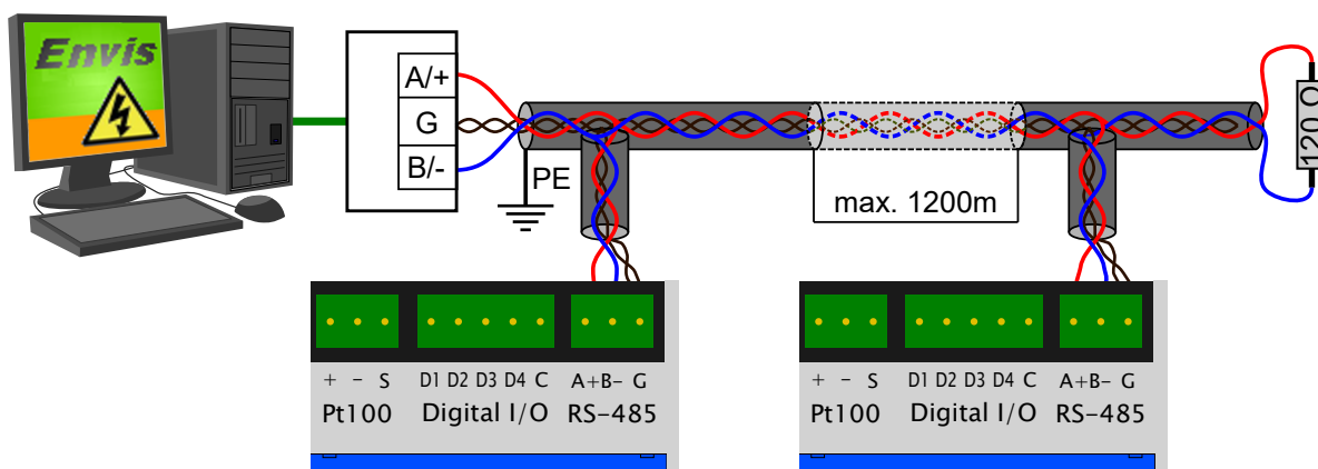
Obrázek 8: Zapojení komunikačních linek sběrnice RS-485 přístrojů ARTIQ 233.
