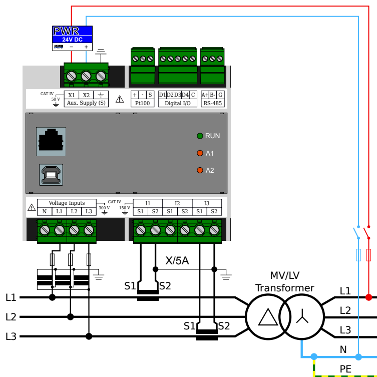
Obrázek 7: Příklad typického zapojení přístroje ARTIQ 233 při měření v síti VN, VVN na sekundární straně přístrojového transformátoru.
