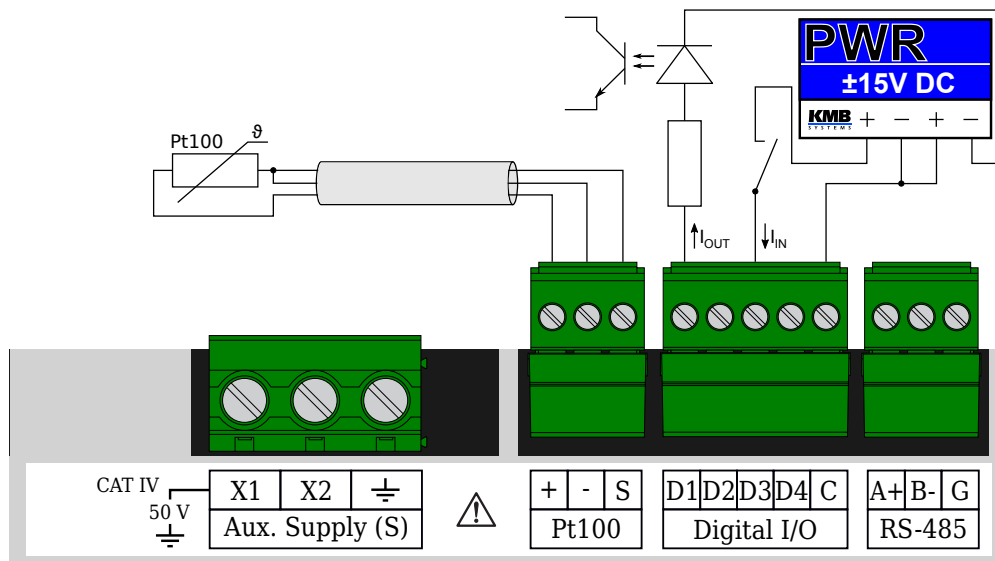
Obrázek 9: Zapojení vstupů a výstupů v přístroji ARTIQ 233.
