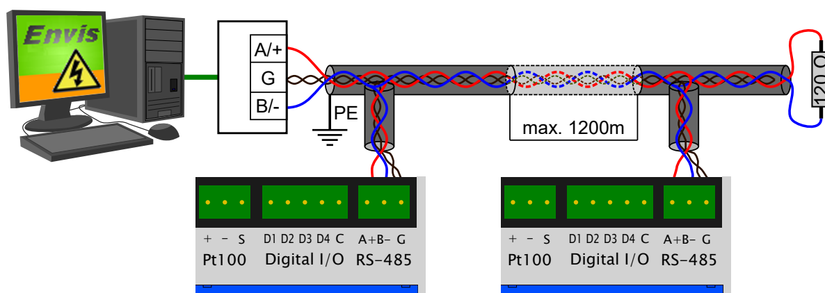
Obrázek 8: Zapojení komunikačních linek sběrnice RS-485 přístrojů SMC 233.
